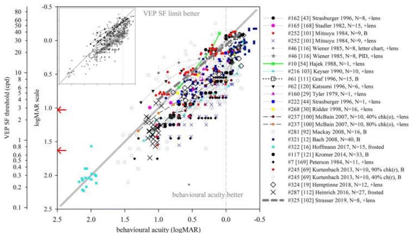
Figure 23 Limite de la fréquence spatiale du PEV (VEP SF) par rapport à l'acuité visuelle comportementale chez des adultes sains, avec une acuité visuelle réduite artificiellement ; la légende indique l'étude, le nombre de sujets (N) et les moyens de réduire l'acuité visuelle ; la ligne grise continue représente l'égalité ; les lignes reliant les symboles représentent les sujets individuels s'ils sont connus, ou bien les données moyennes d'un même groupe de sujets ; les flèches rouges sur l'axe SF indiquent les damiers 60' (0,71 cpd) et 15' (2,8 cpd) ; Hamilton et al., VEP estimation of visual acuity : a systematic review , 2021 (72)
